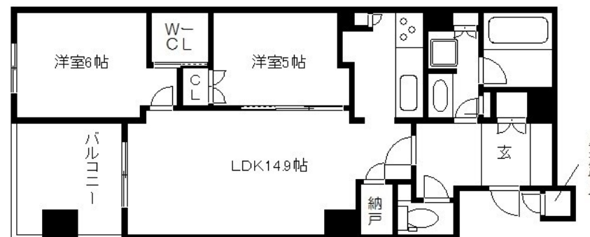
【間取り図】
